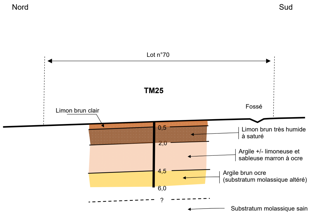
Schéma indicatif ( \approx 1/200 )
