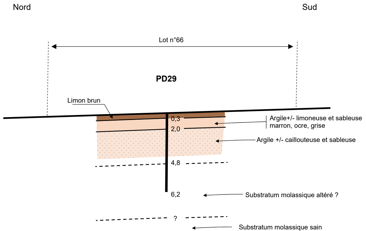
Schéma indicatif (≈ 1/200)
